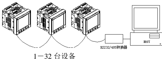
RS-485 总线链接示意图
