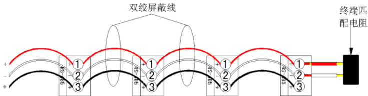
网络链接示意图
