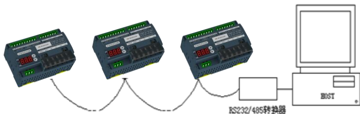
通讯接线示意图
